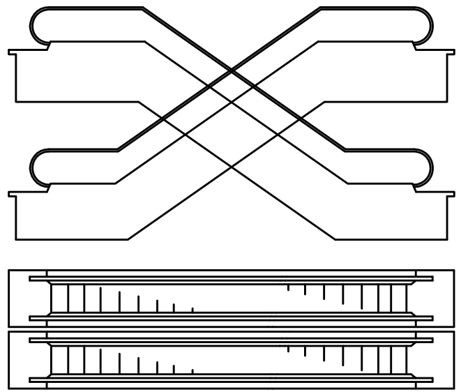
Перекрестное расположение
