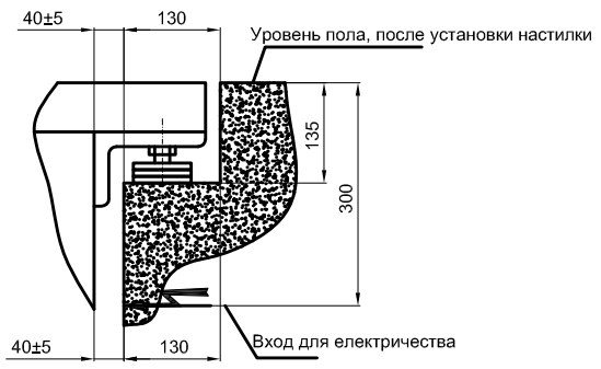
Параллельное расположение
